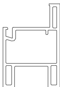
Marco Hoja Móvil. Sup PD130 61113EKO000
