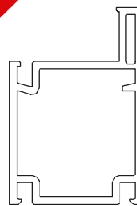
Hoja Móvil Lateral PD130 61112EKO000
