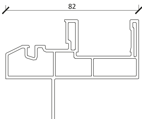
Marco Americana EKO82 61101EKO000
