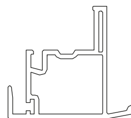
Traslapo Móvil EKO82 61103EKO000
