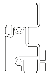
Traslapo Fijo EKO82 61104EKO000
