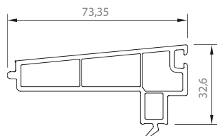
61474VER Tapa Traslapo INOVA
